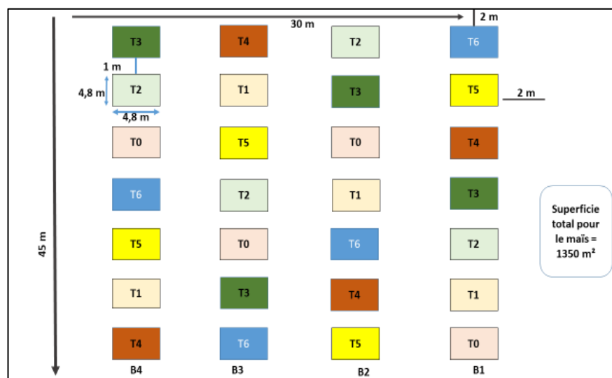
Figure 2. Dispositif expérimental
