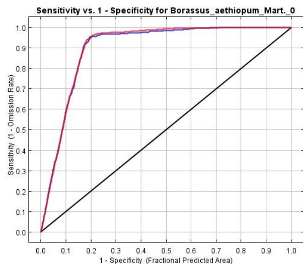
Figure 4: Valeur de l'aire sous la courbe (AUC, Area Under Curve)
