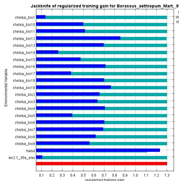
Figure 3: Contribution des variables bioclimatiques : test de test Jackknife.
